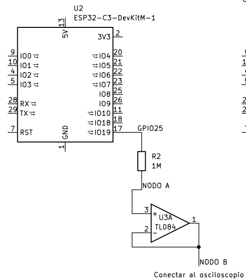
Corrección con buffer TL084
