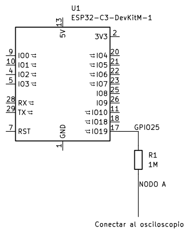
Efecto de carga (sin buffer)
